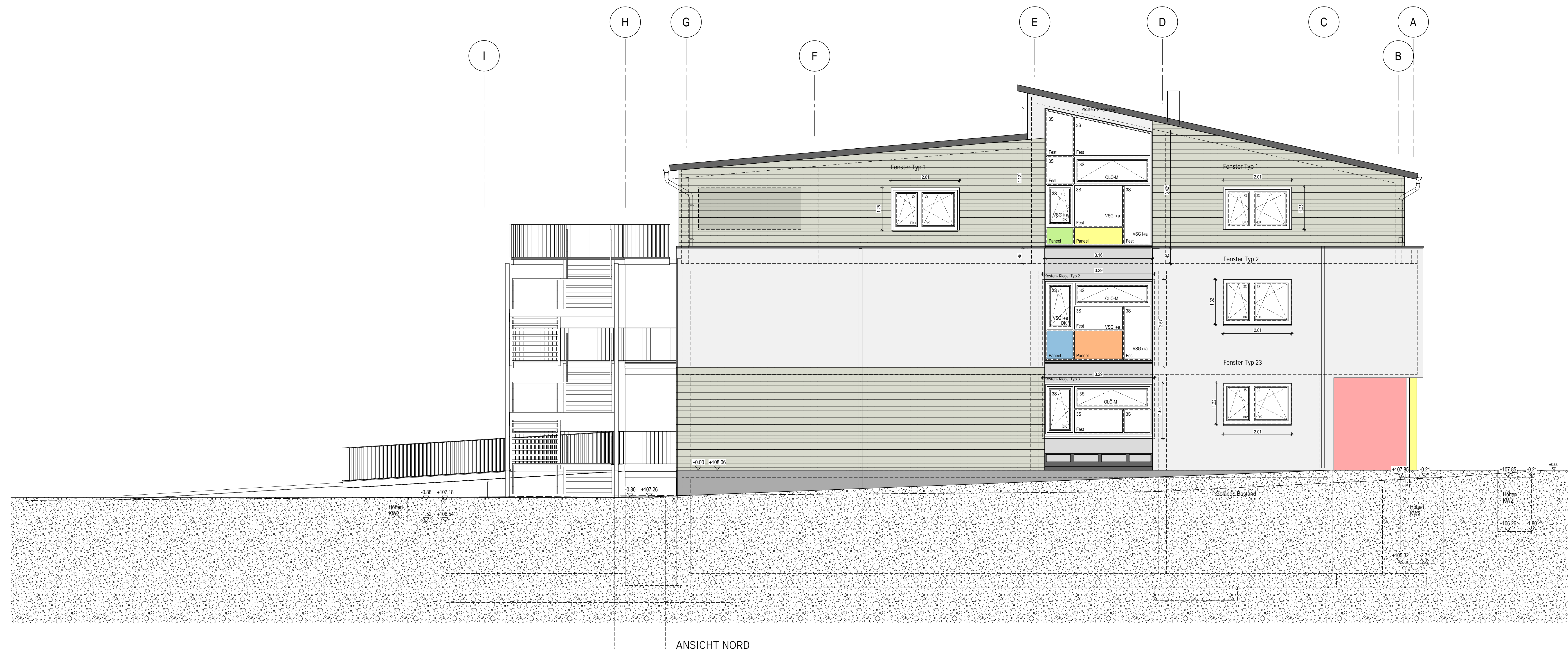
ANSICHT NORD
